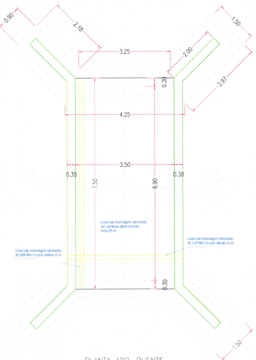
PLANTA ARQ. PUENTE ESC: 1/20
